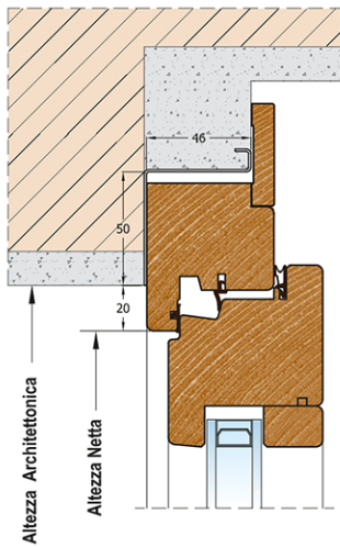
3. Sezione verticale - Nodo superiore
