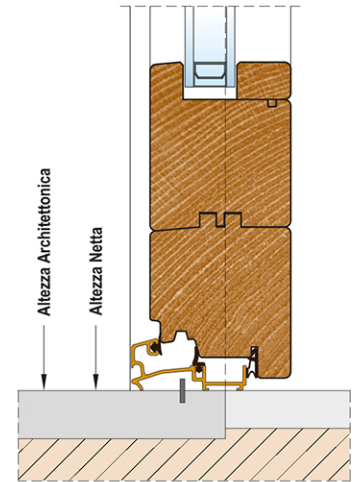
6. Sezione verticale Nodo inferiore porta-finestra
