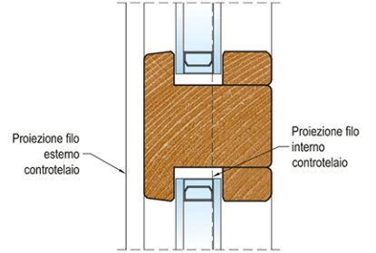
5. Sezione verticale Nodo centrale porta-finestra
