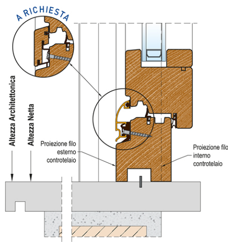
4. Sezione verticale - Nodo inferiore finestra
