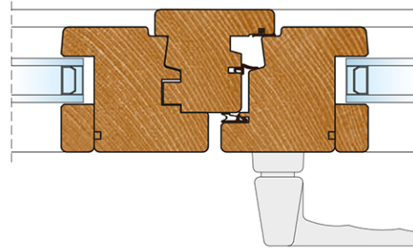
2. Sezione orizzontale - Nodo centrale
