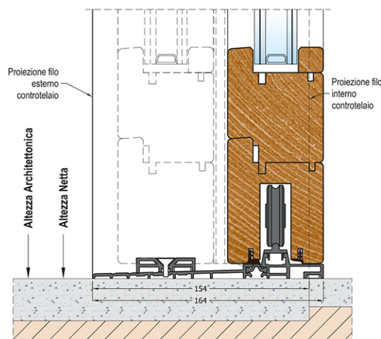
5. Sezione verticale - Nodo inferiore finestra e porta-finestra
