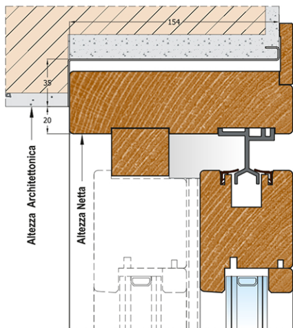
4. Sezione verticale - Nodo superiore
