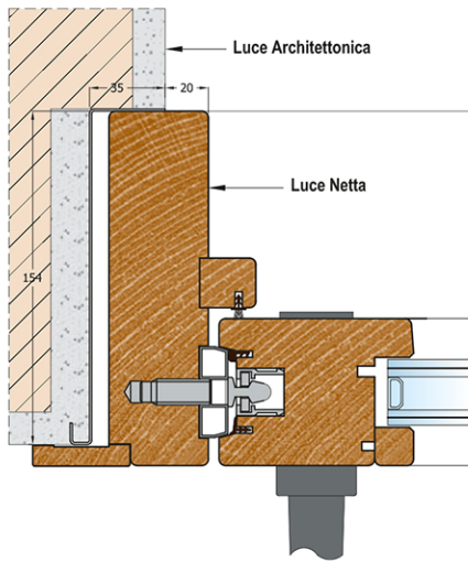
4. Sezione verticale - Nodo superiore
