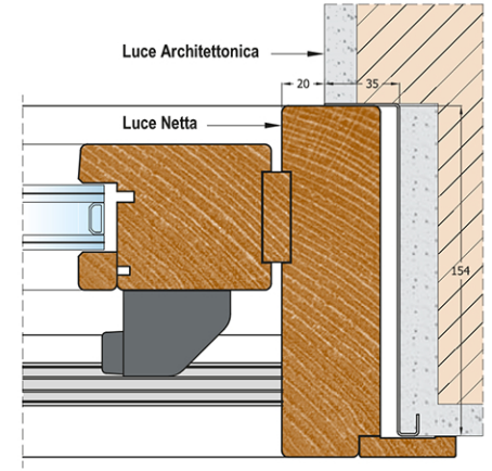
3. Sezione orizzontale - Nodo laterale
