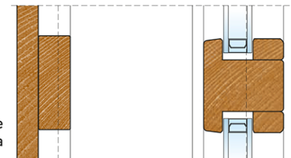
5. Sezione verticale Nodo centrale porta-finestra
