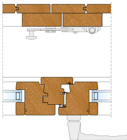
2. Sezione orizzontale - Nodo centrale
