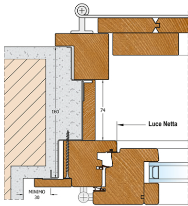
1. Sezione orizzontale - Nodo laterale
