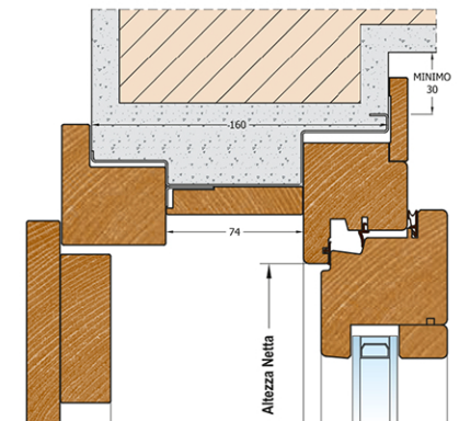
3. Sezione verticale - Nodo superiore
