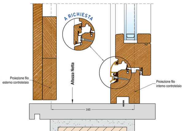
4. Sezione verticale - Nodo inferiore finestra
